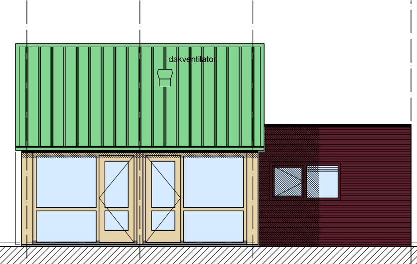
OOSTGEVEL
