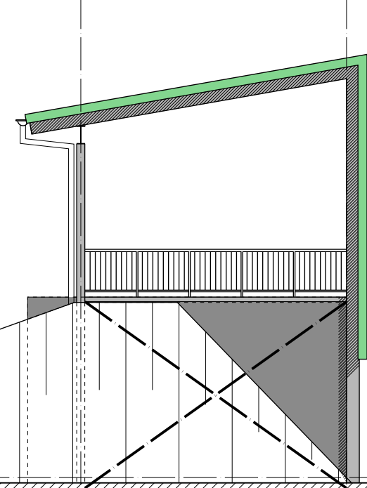
WESTGEVEL
