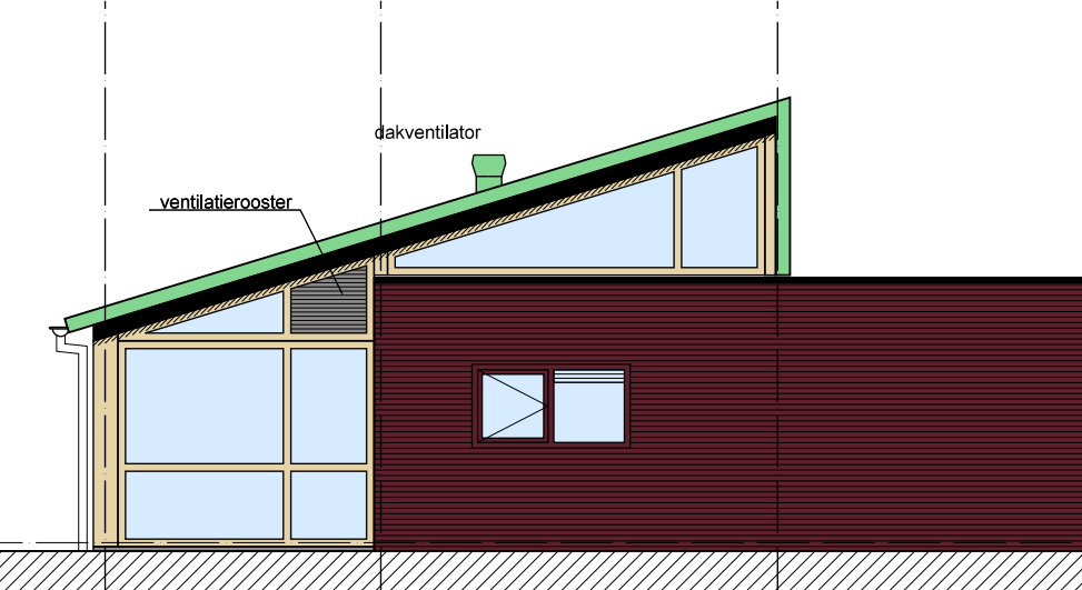
NOORDGEVEL
