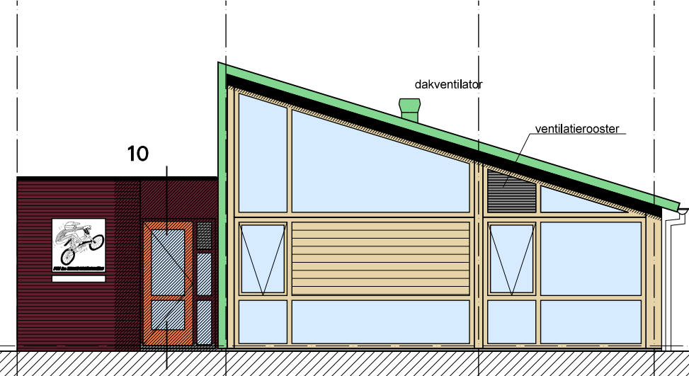
ZUIDGEVEL
