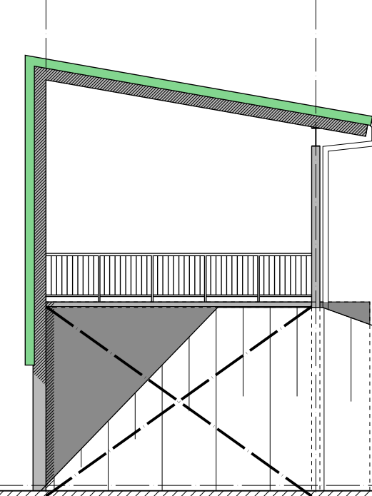
OOSTGEVEL
